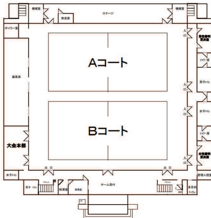
西部体育館平面図（1F）
